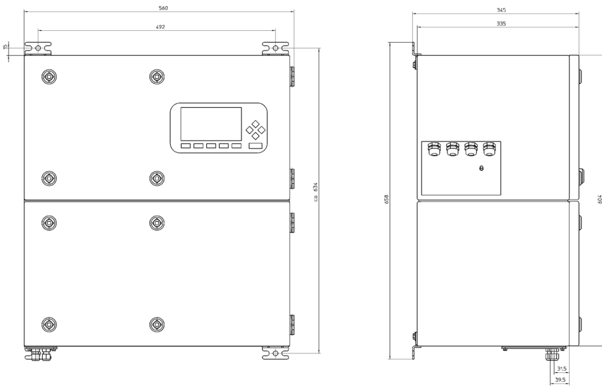
Zweiteiliges Gehäuse
