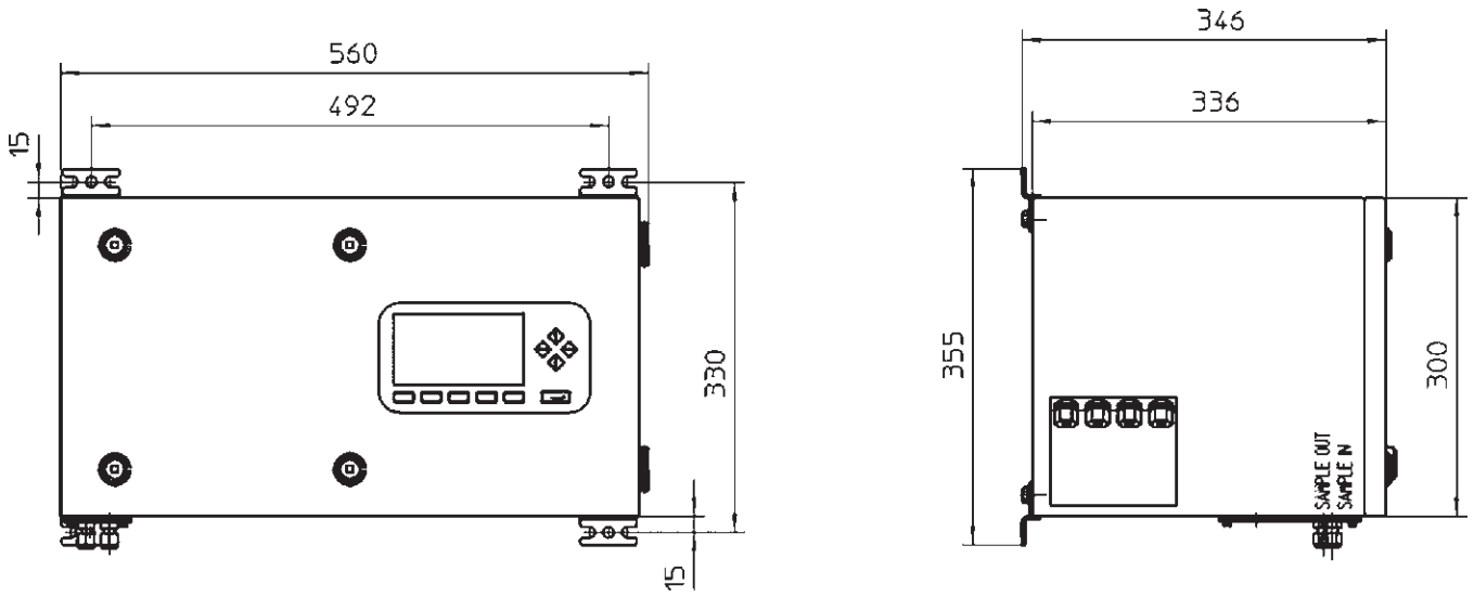
Einteiliges Gehäuse
