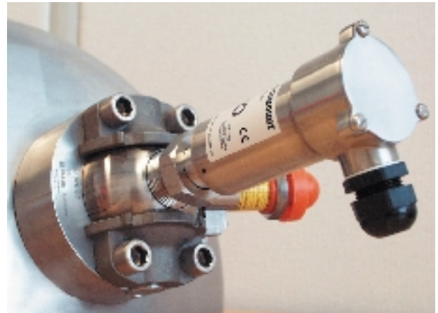
Uusi mittausratkaisuvaihtoehto: Rosemount 1810 paine- ja pintalähetin tuttuihin PASVE ja G1”-asennuksiin
