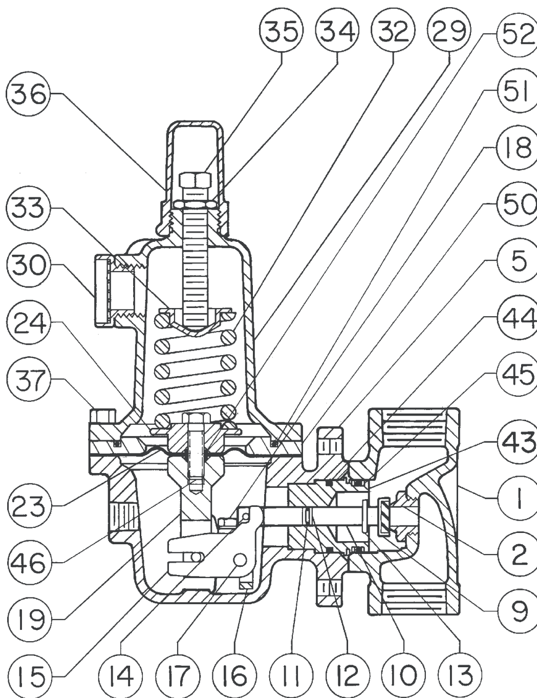
Ilustracja 12. Schemat budowy regulatora typ 627HM
