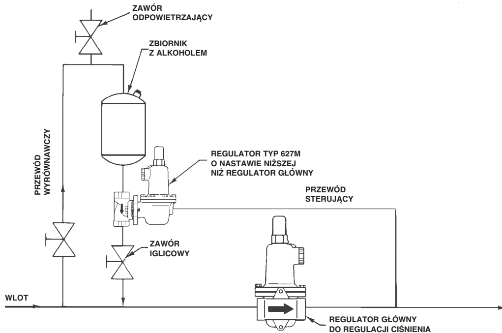
Ilustracja 3. Schemat systemu przeciwooblodzeniowego
